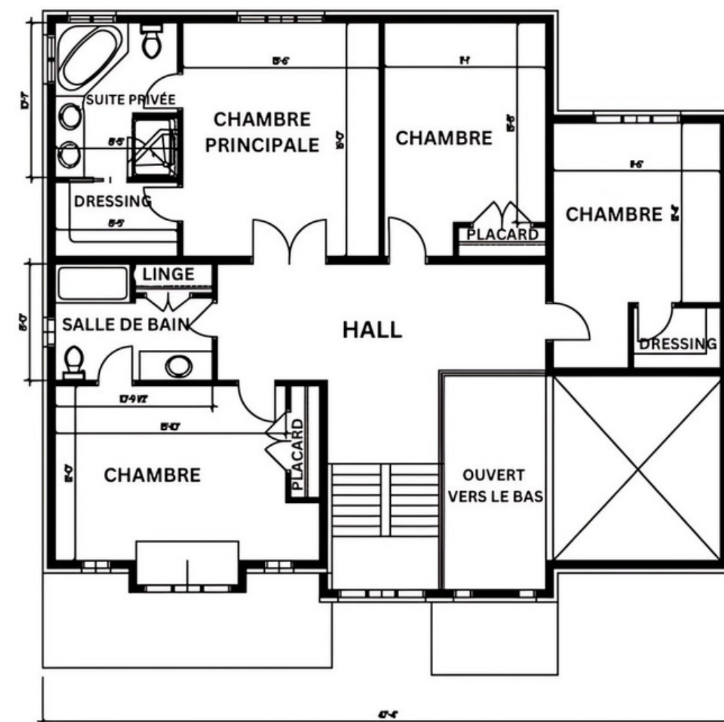
PLAN DU 2 e ÉTAGE 1385 PI 2
