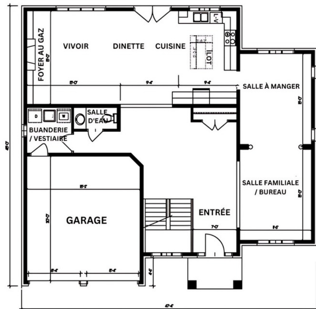
PLAN DU REZ-DE-CHAUSSÉE 1502 PI 2
