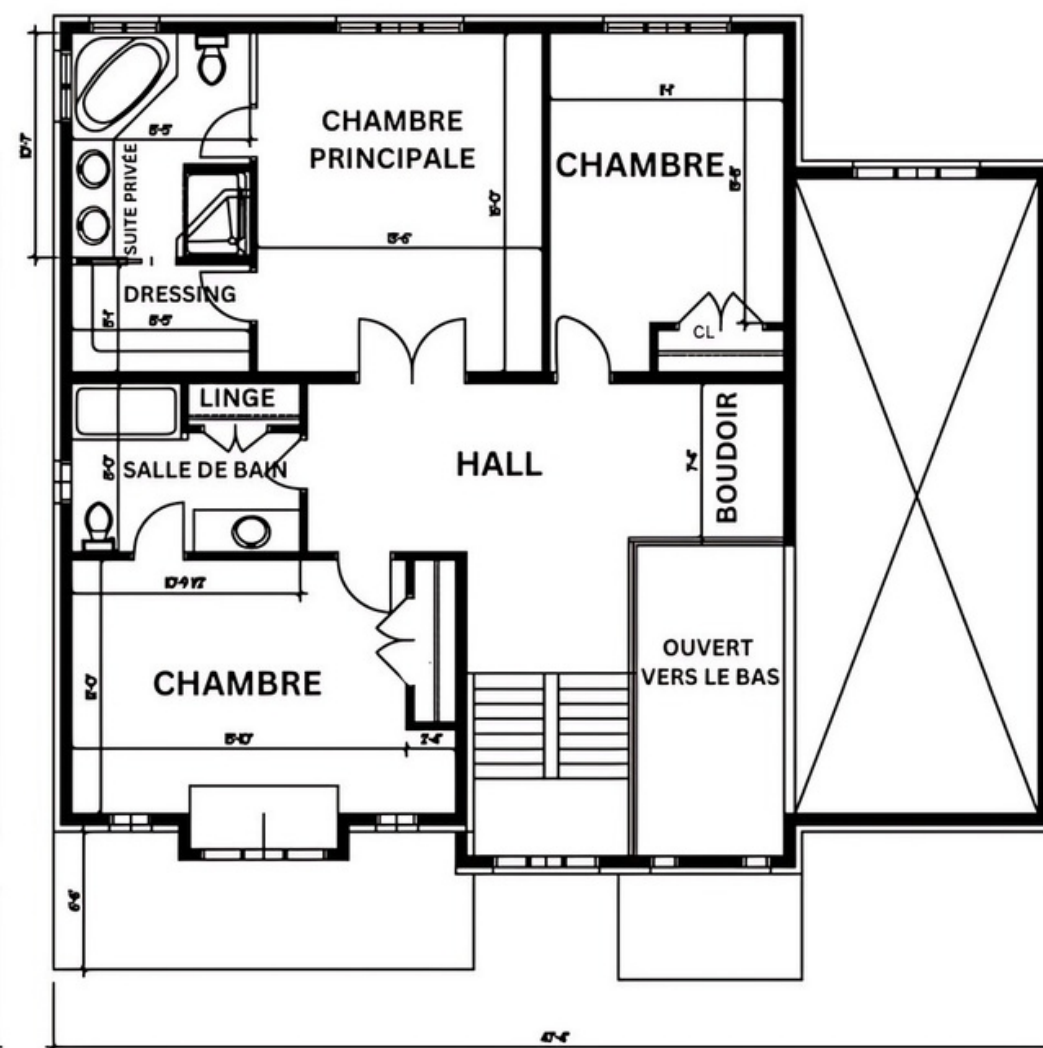
PLAN DU 2 e ÉTAGE 1160 PI 2
